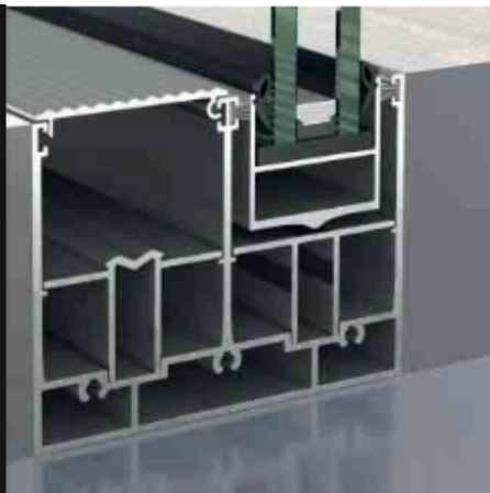
ASS 39 PD.NI Sliding System ASS 39 PD.NI
