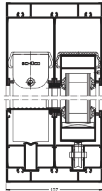
Vertikalschnitt, Schüco Schiebesystem ASS 39 PD.NI, Maßstab 1:3
